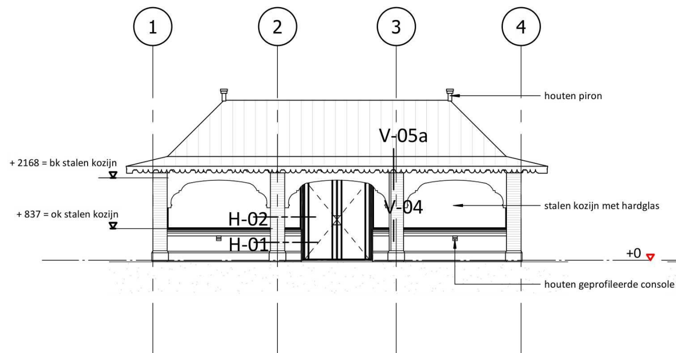
voorgevel
