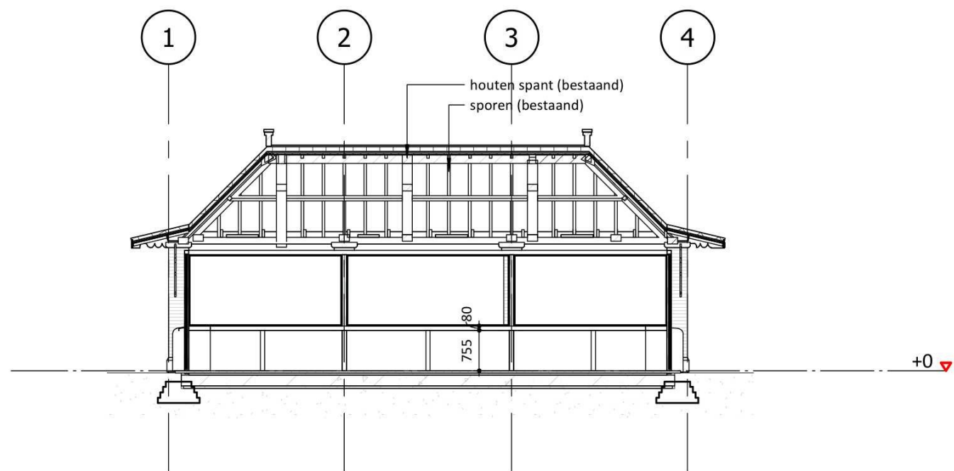
doorsnede A
