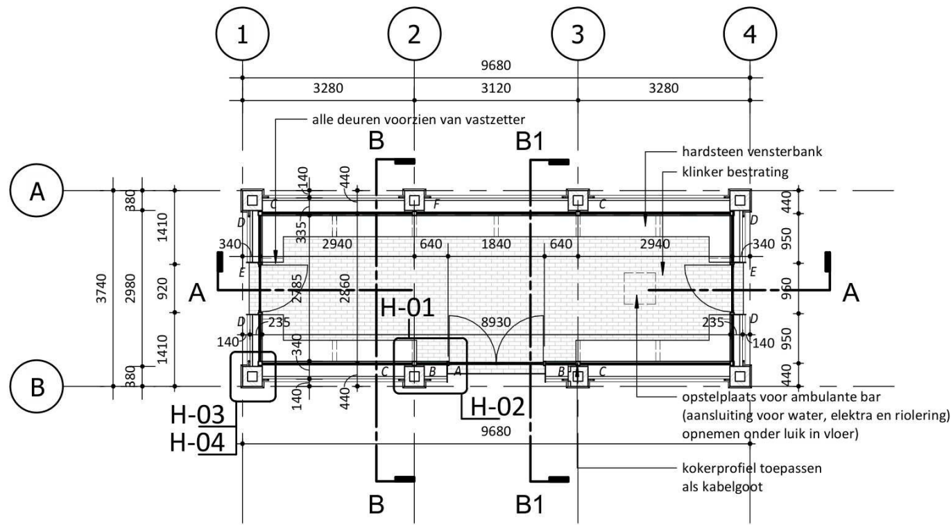
begane grond
