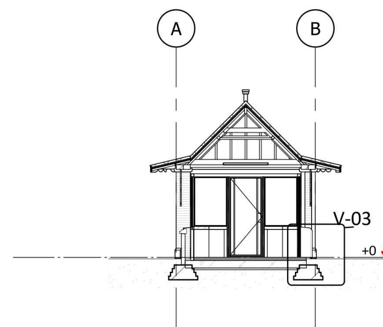
doorsnede B1
