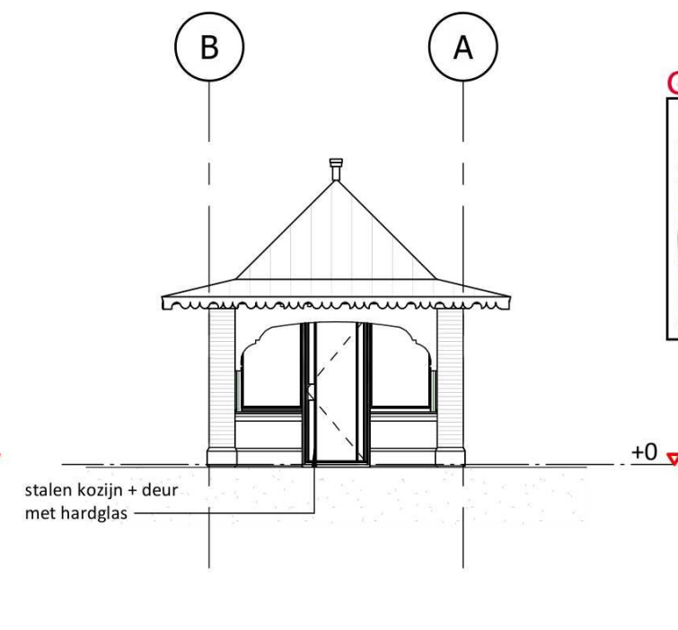
rechtergevel
