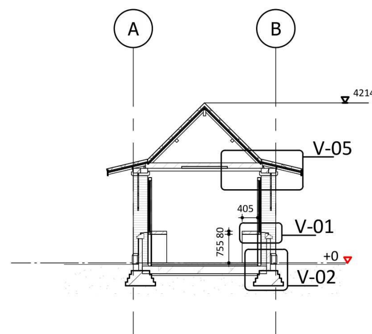
doorsnede B
