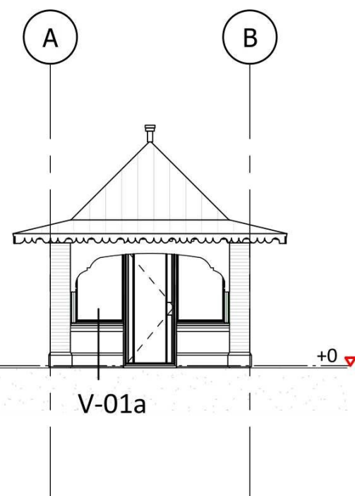
linkergevel
